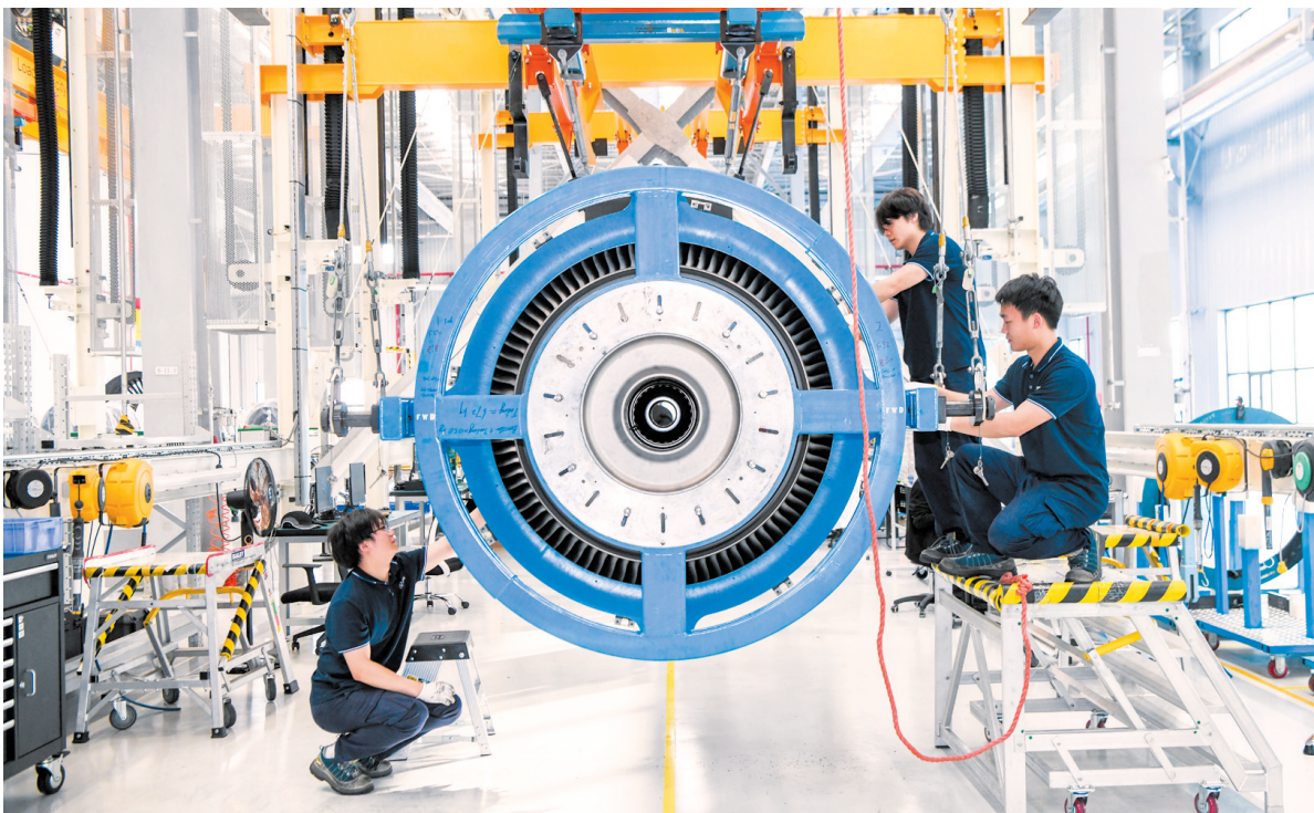
▲近日,在位于海口空港综保区的海口美兰三空港吉耐斯航空发动机维修工程有限公司,工作人员正在检修航空发动机。本报记者 苏磊坤 实习生 陈新锐 摄
